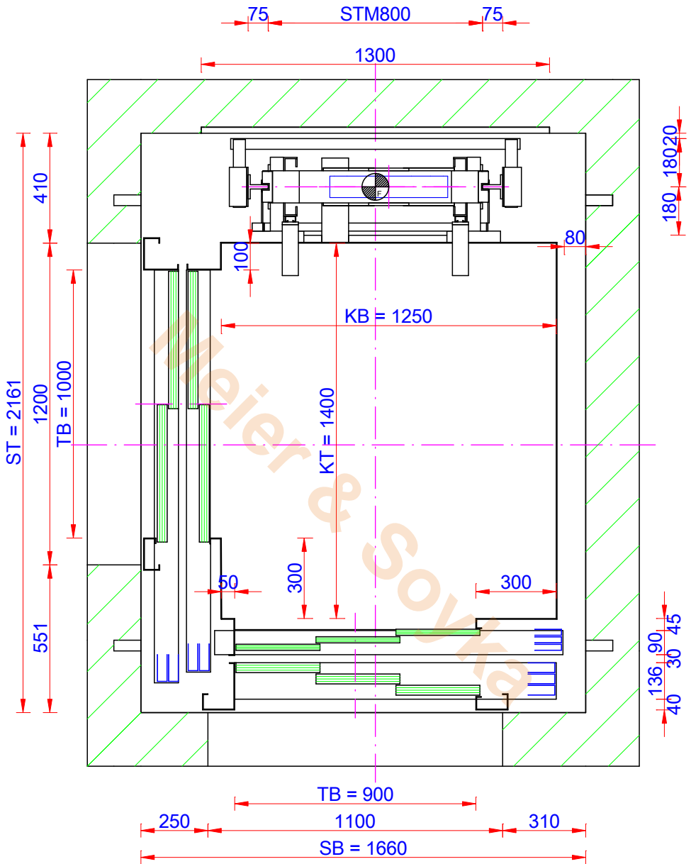
Schachtgrundriss Maßstab: 1:20
