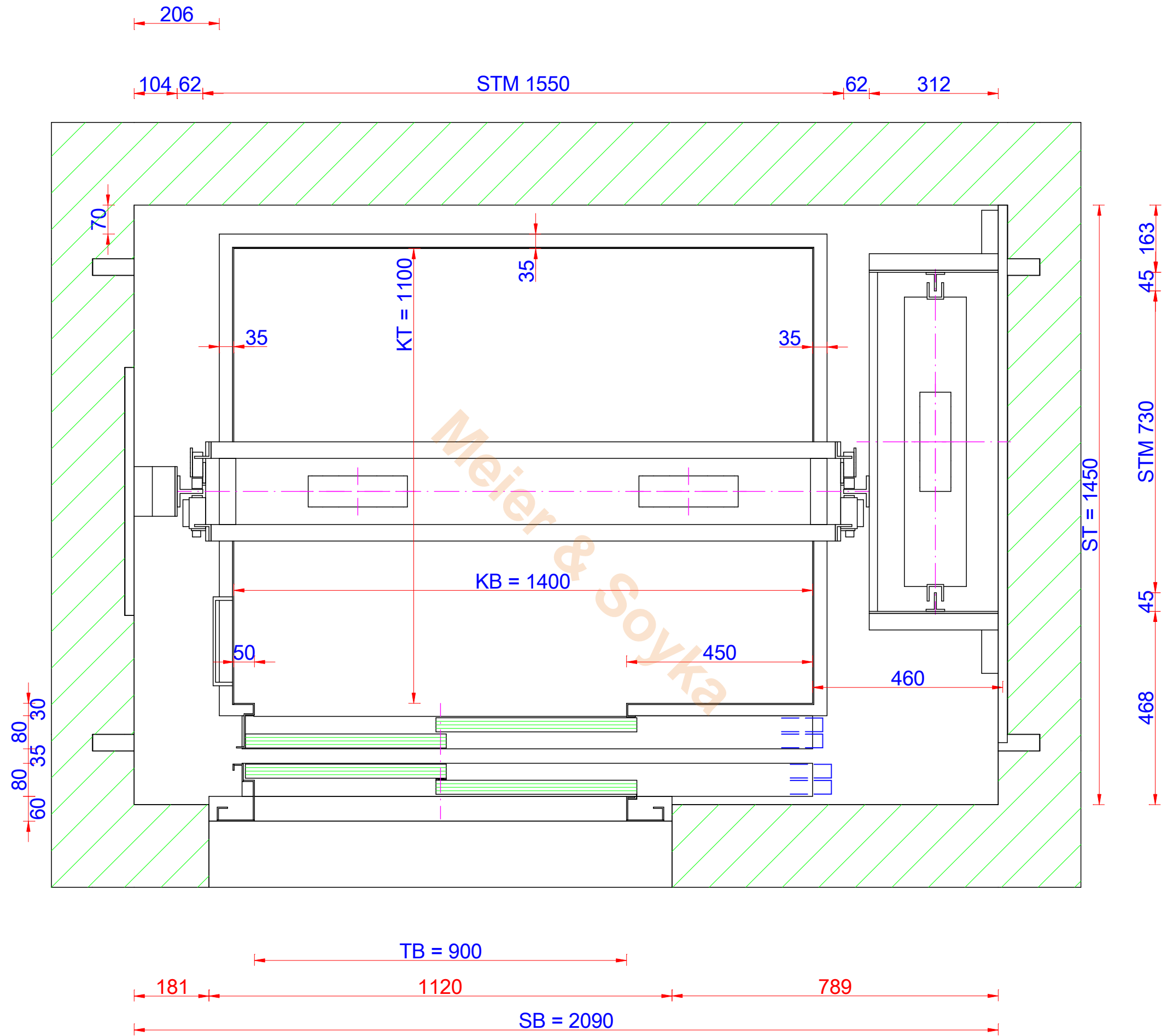
Schachtgrundriss Maßstab: 1:10
